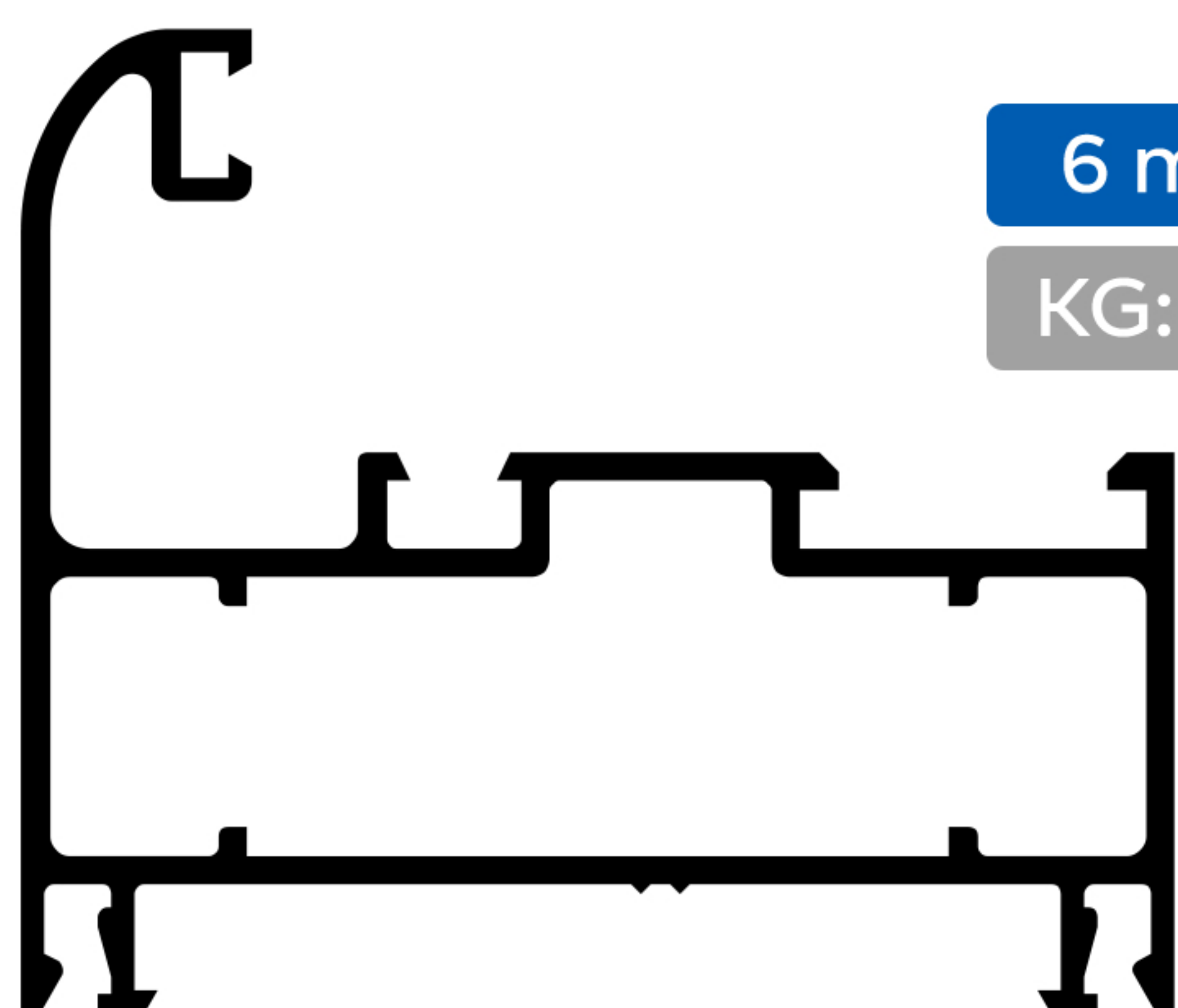
B Marco P/Fijo Y Ventana De Abrir Atp - Cod. 3055
