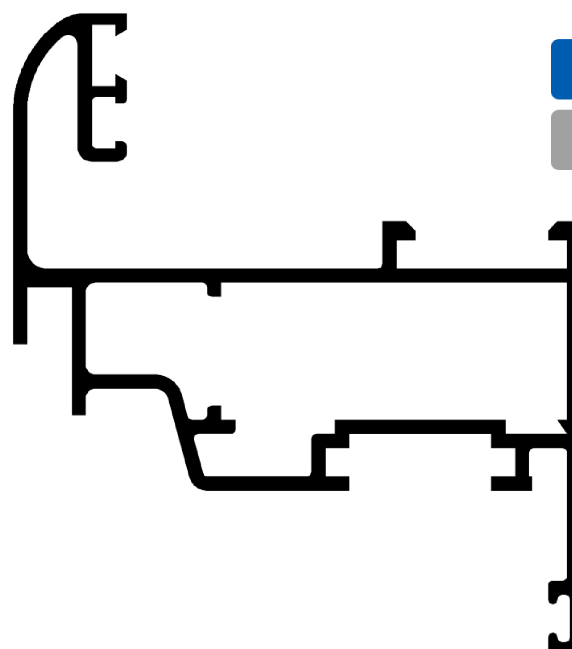
B Hoja Curva Ventana De Abrir Atp - Cod. 3052
