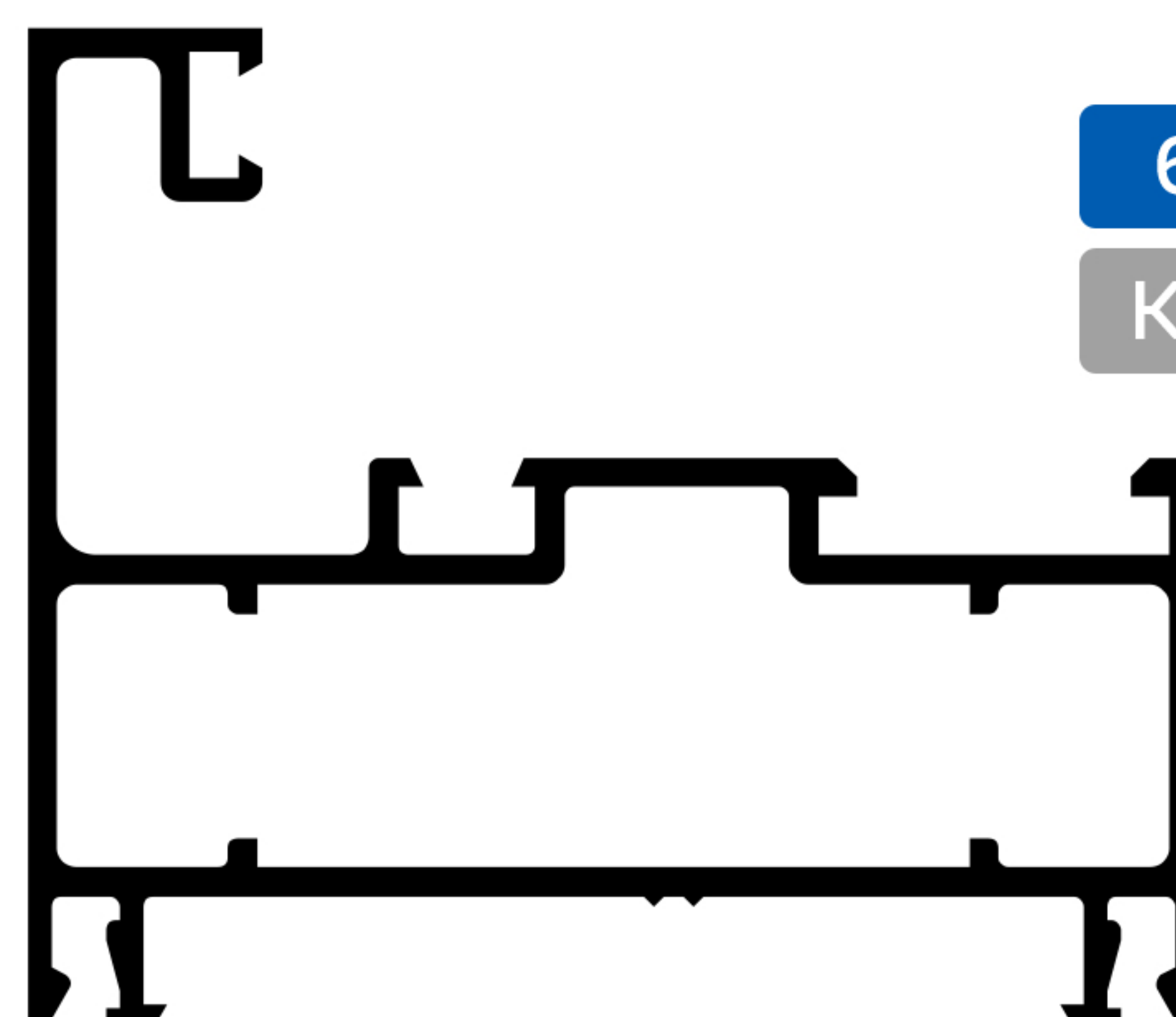
B Marco Paño Fijo Recto Atp - Cod. 3059
